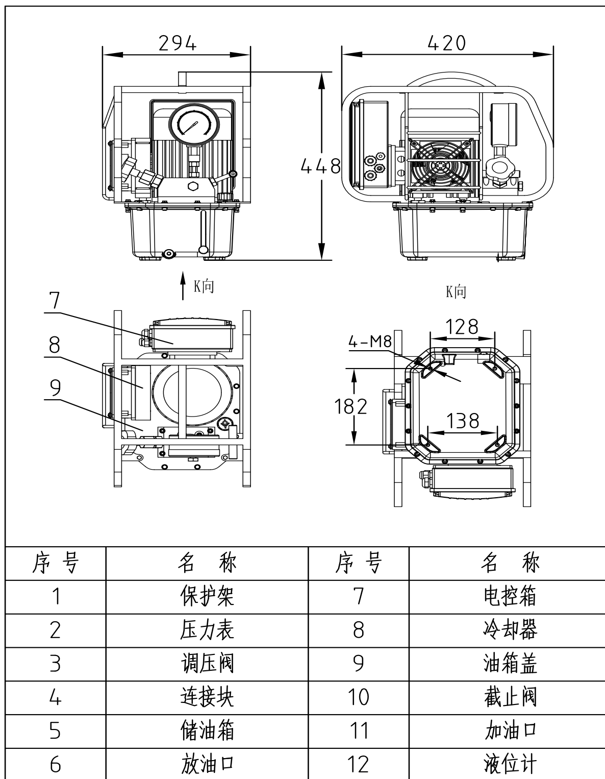
装配示意图
