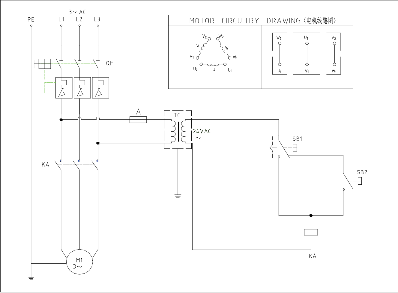
HMP系列液压泵电路控制原理图(三相220V)
