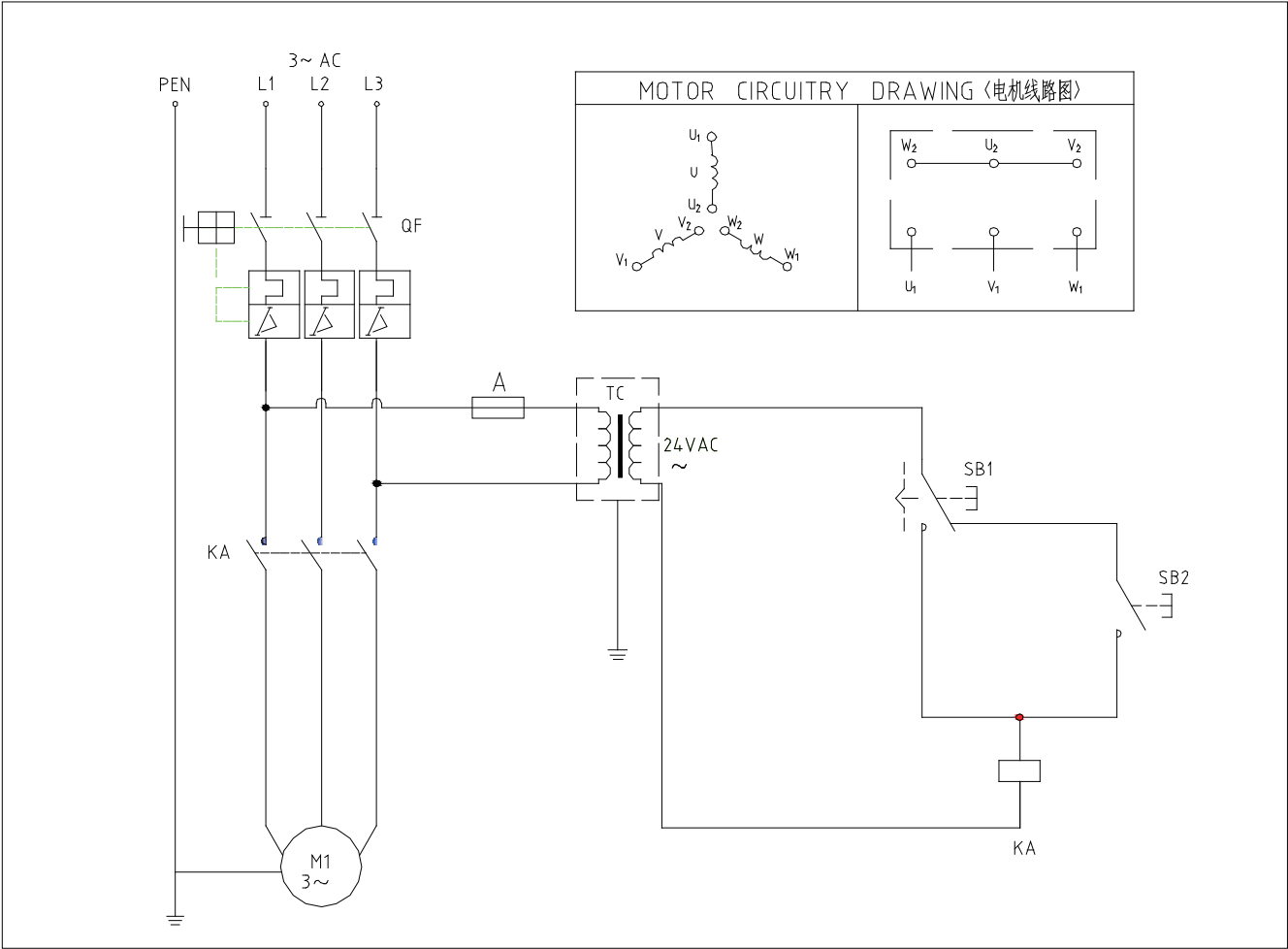
HMP系列液压泵电路控制原理图(三相380V)
