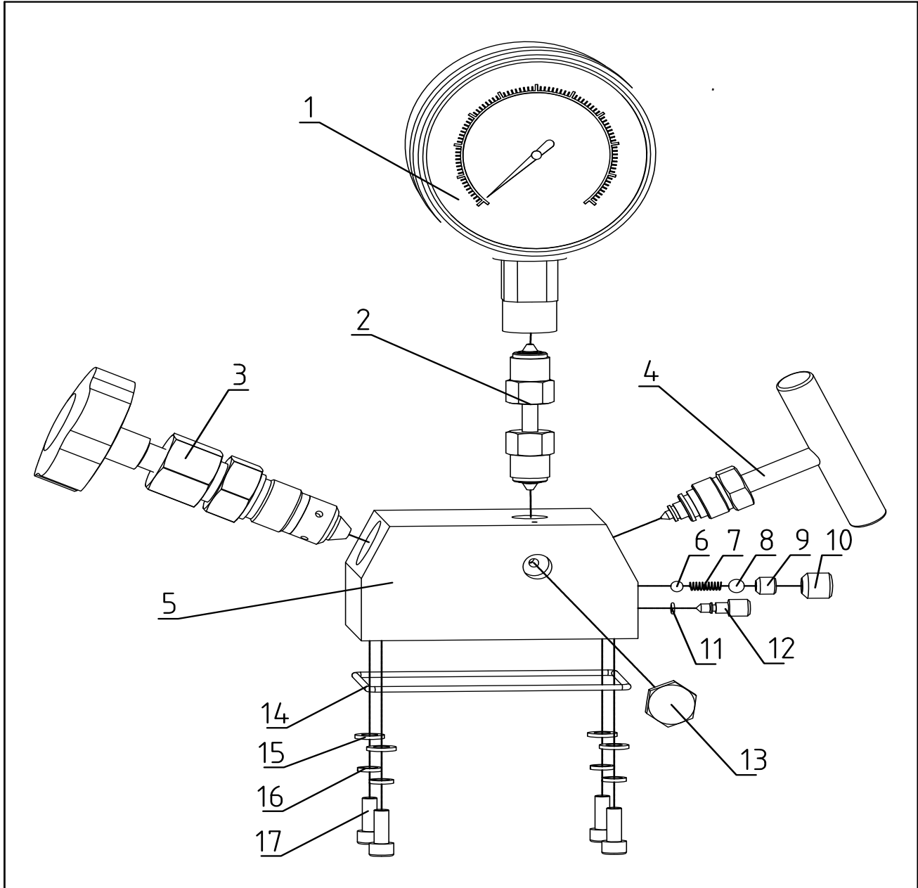
泵阀组模块爆炸图
