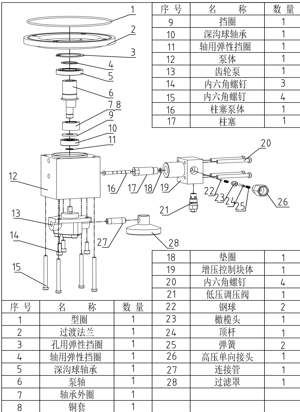
HMP系列泵体模块爆炸图
