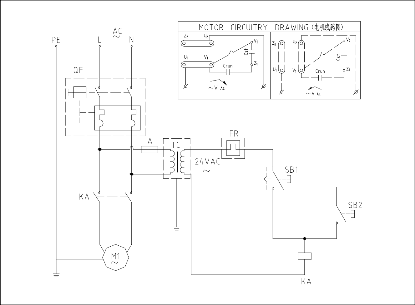
HMP系列液压泵电路控制原理图(单相220V)
